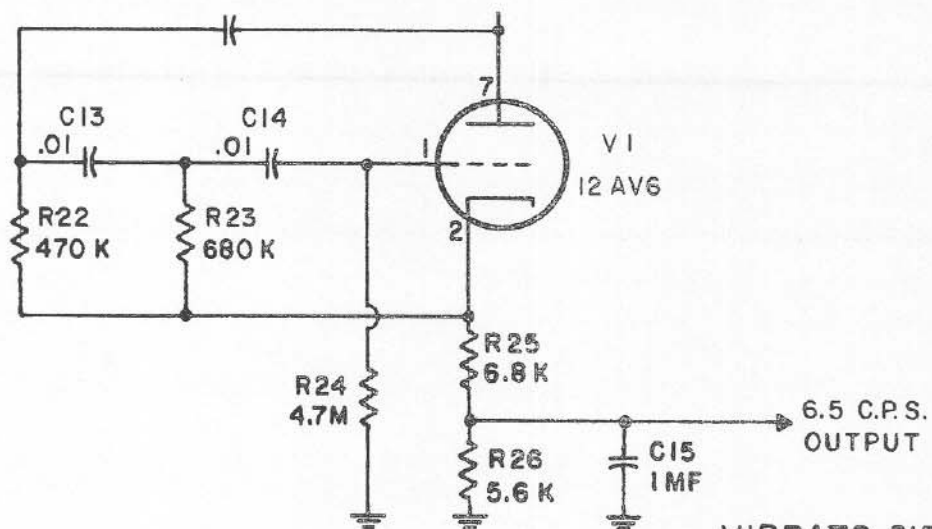
VIBRATO CIRCUIT
